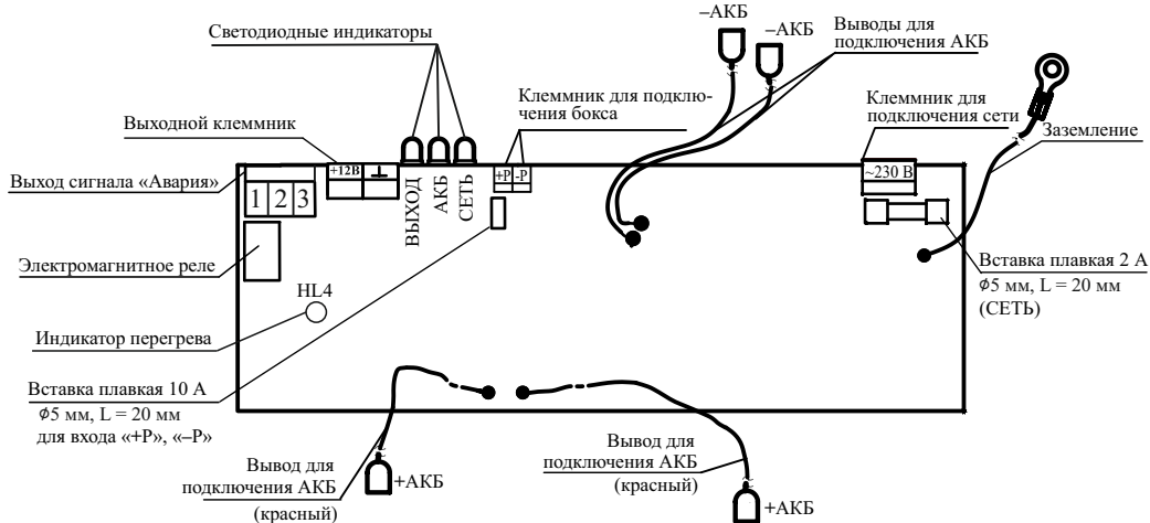
Рисунок 1 – Плата источника
