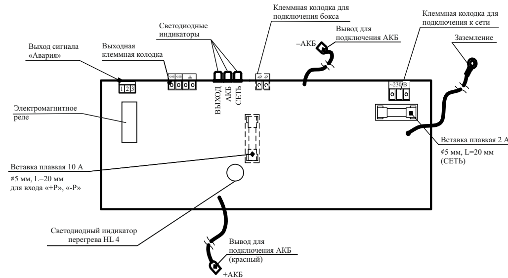
Рисунок 1 – Плата источника
