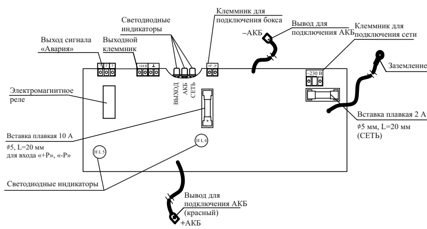
Рисунок 1 – Плата источника
